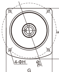
A-出力法兰 A-Output Flange
